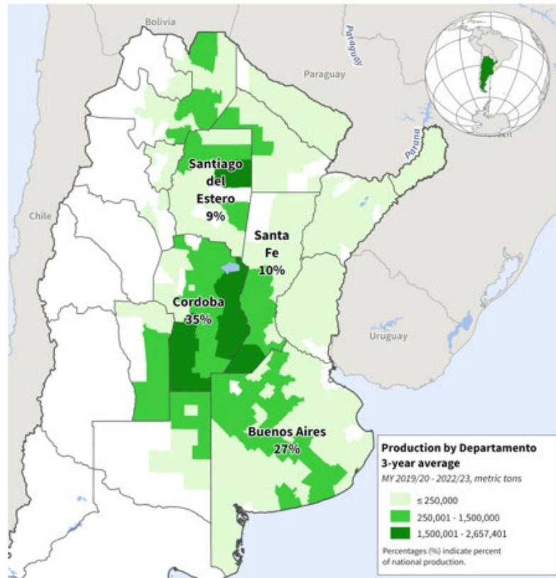
Argentina Corn
